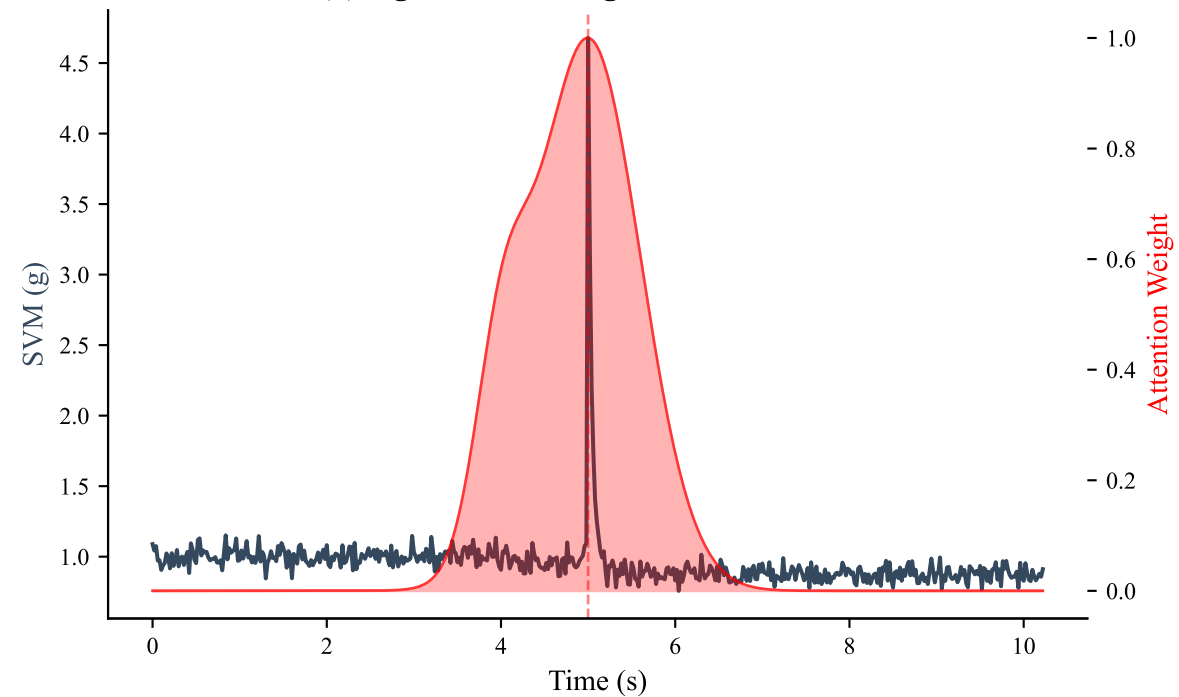
(d) Attention Weight Distribution
