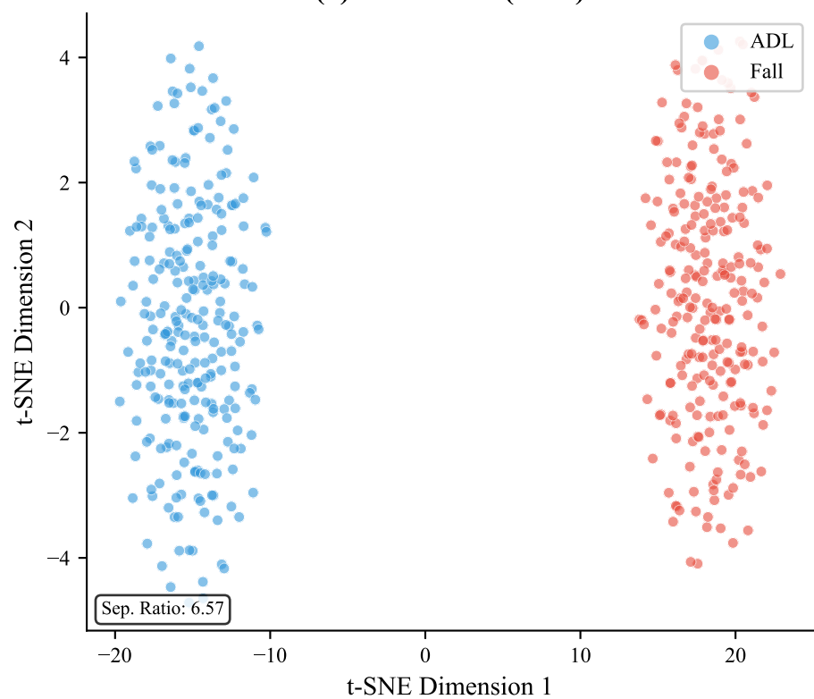
(b) AMSNetV2 (Ours)
