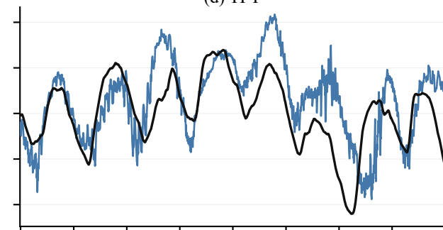
(d) TFT
