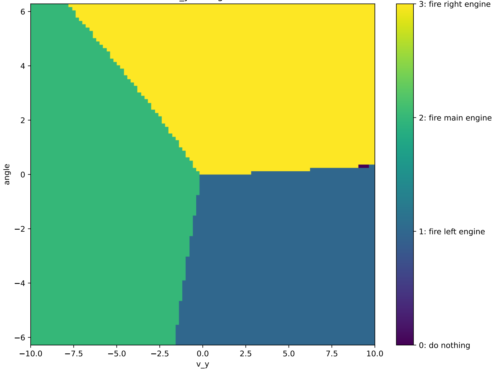
v_y vs angle
