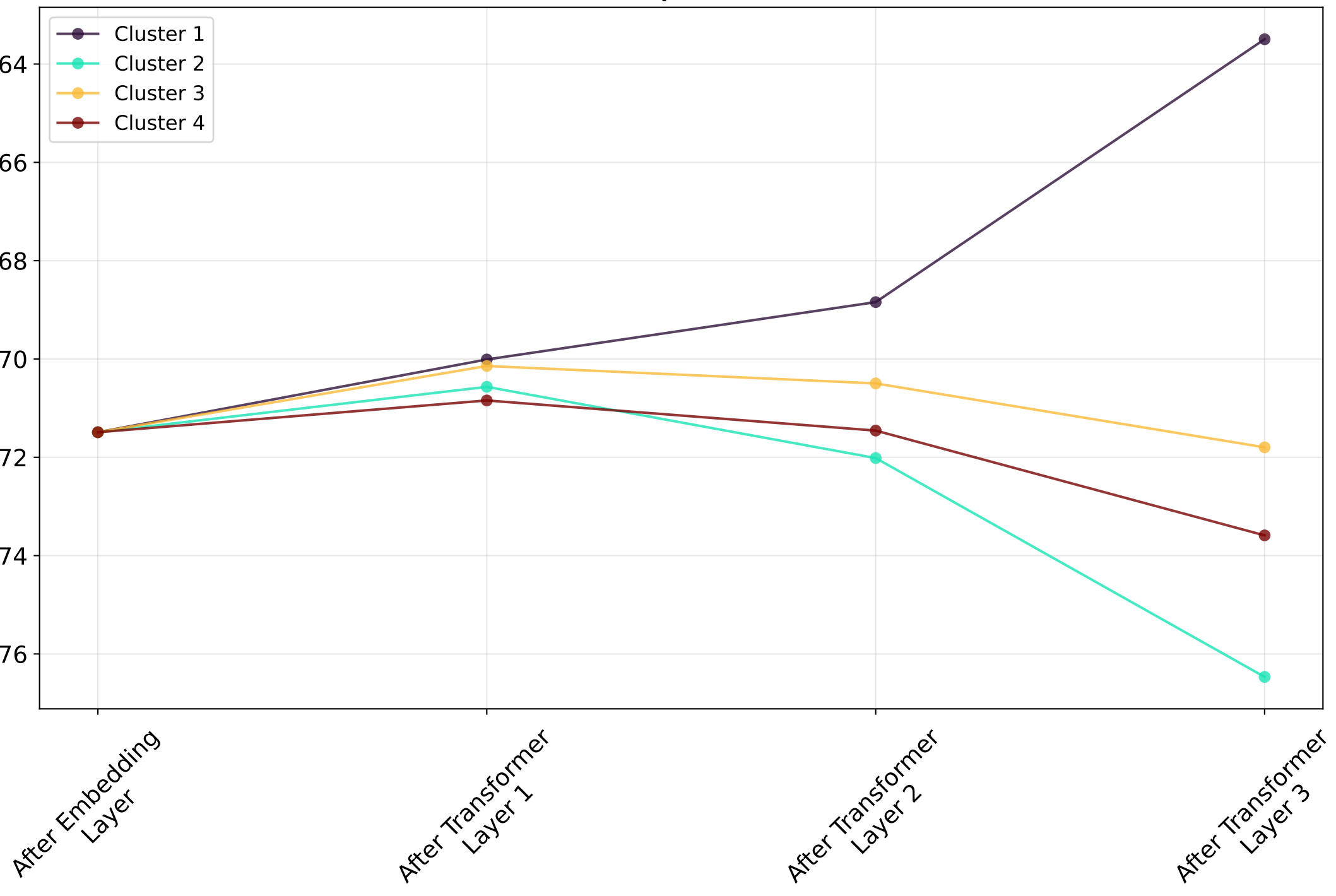
QM9
