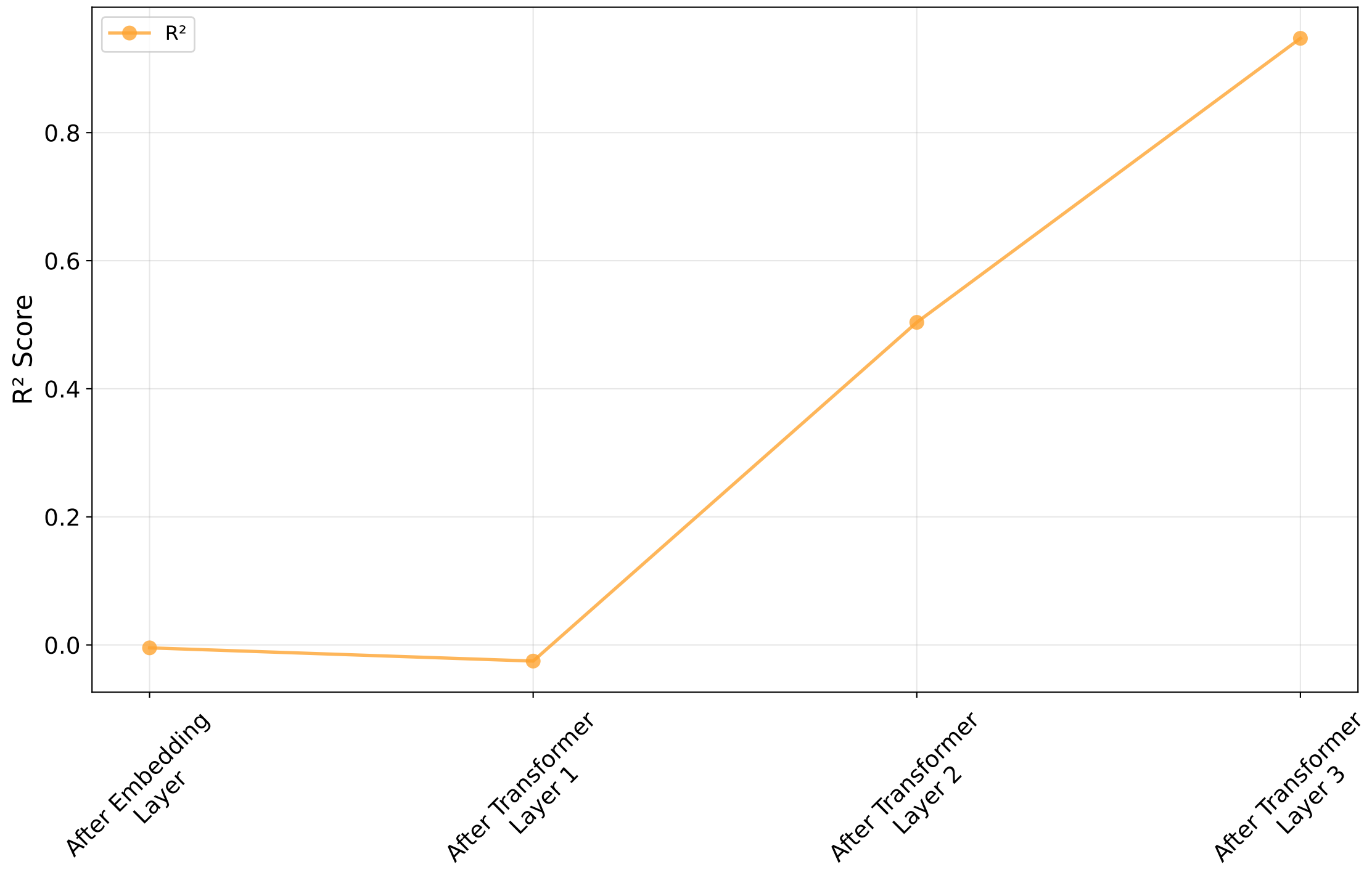
ESOL - R^2
