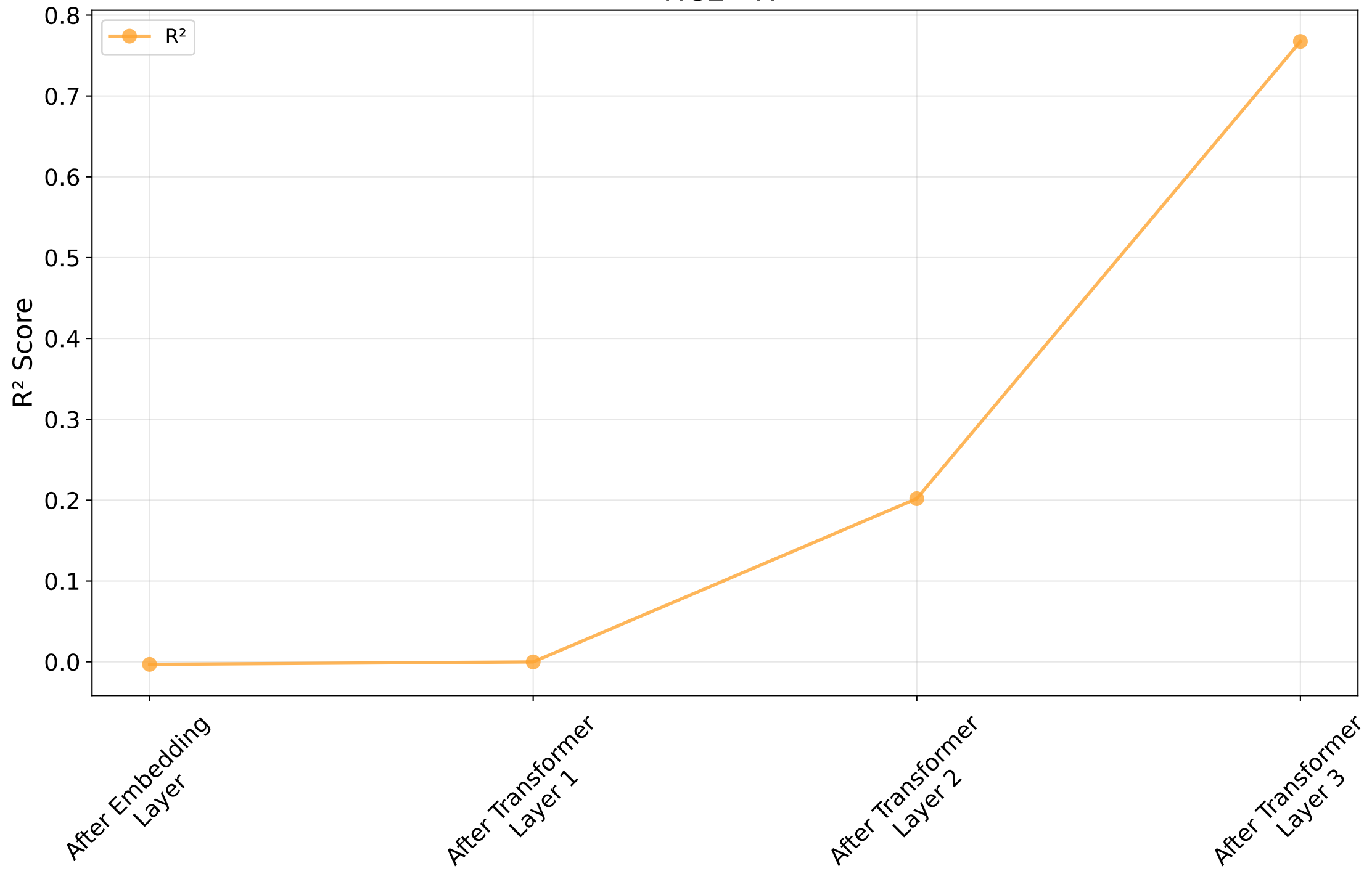
HCE - R^2
