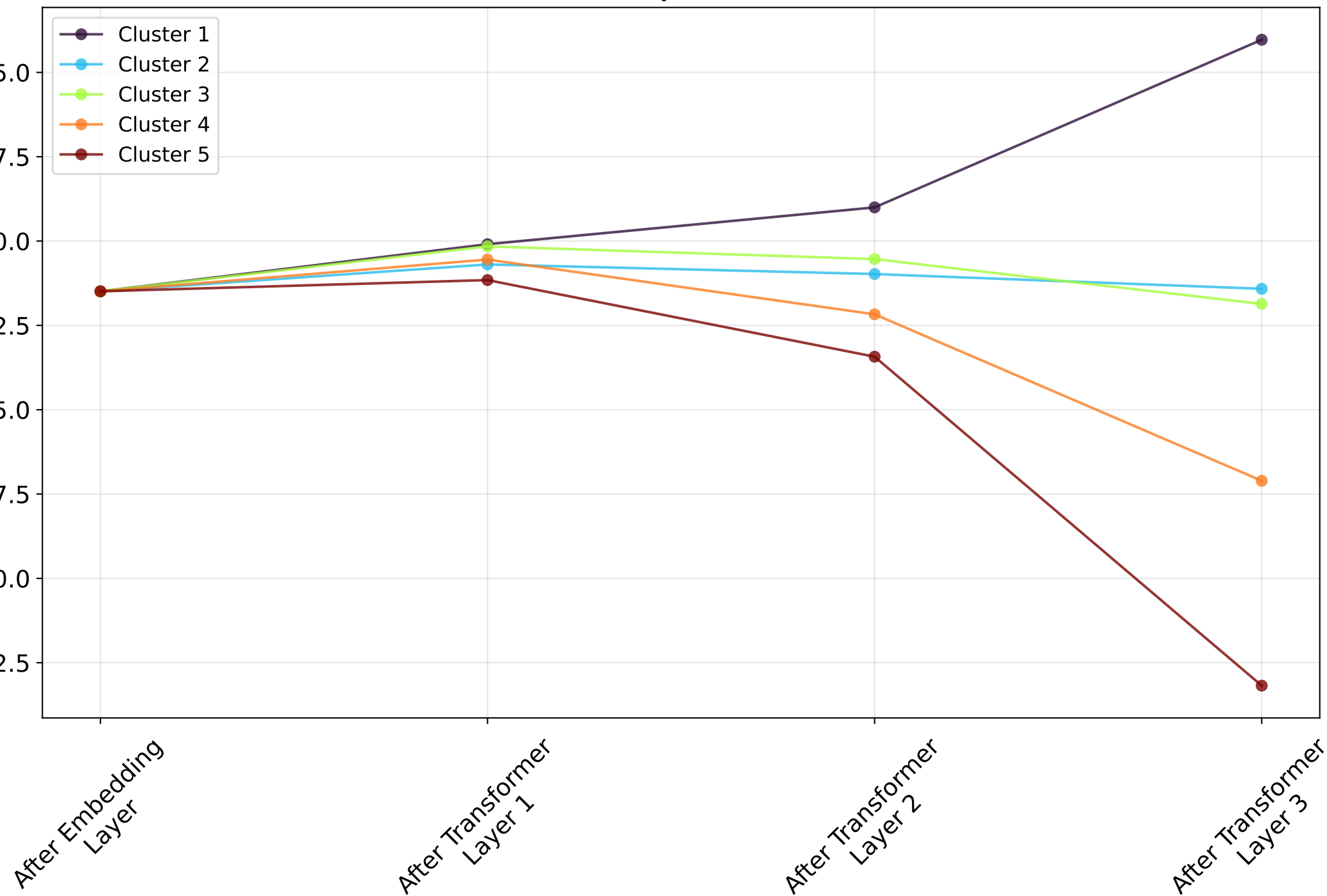
QM9
