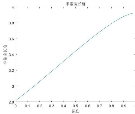
图 12. 统一内聚力相场模型损伤半带宽
