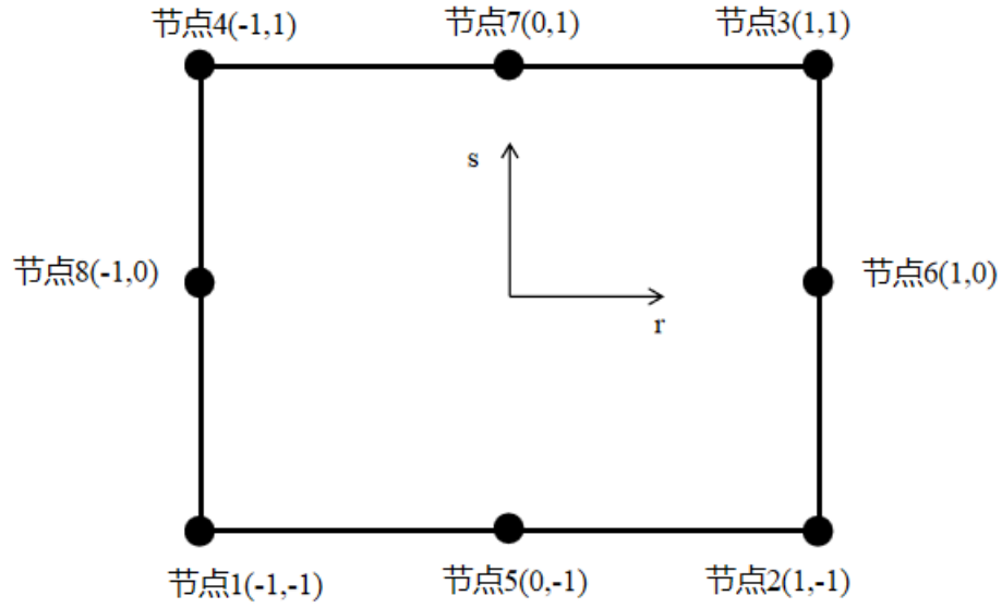
图 7-2 四边形八节点单元示意图
