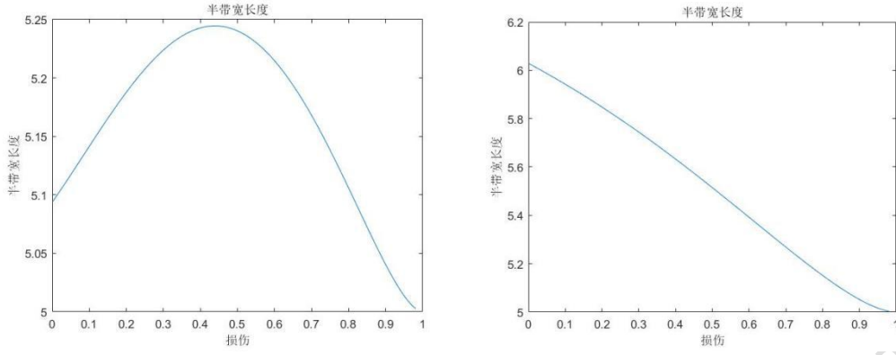
图 13. (3.24)相场模型损伤半带宽 (左: s=1.1 ; 右: s=1.5 )
