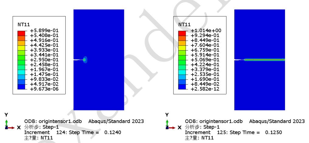
图 7.3 默认收敛条件下的 AT2 相场模型，左图与右图仅相差一个增量步，裂纹即迅速贯穿扩展，在此增量步内经历了多轮迭代
