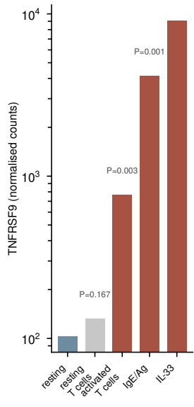
c 4 donors, paired (GSE235240)
