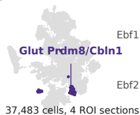
a UMAP
