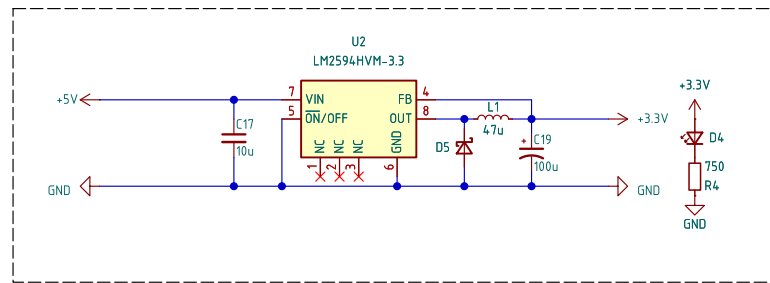
Питание 3.3В
