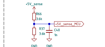
Измерение +5V
