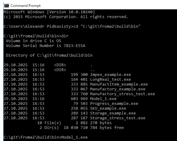
Рисунок 13 Запуск программы Model 1
