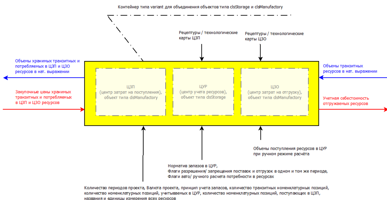
Рисунок 31 Принципиальная схема модели склада с двумя центрами затрат на базе класса clsAgregate
