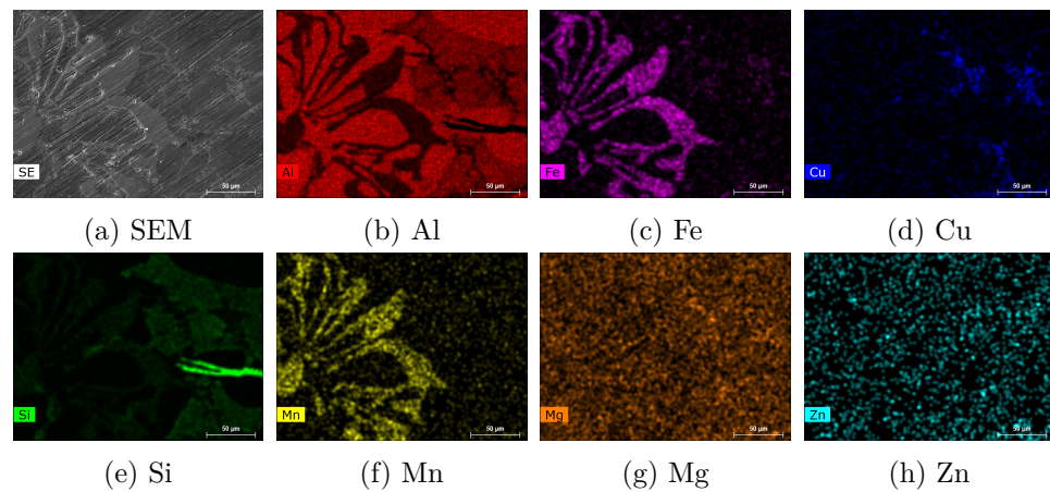
Figure 4.1: Pannel comparativo SEM-EDS em disposição compacta de 2x4.
