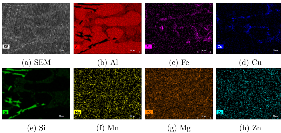
Figure 4.2: Paineil comparativo SEM-EDS em disposição compacta de 2x4.
