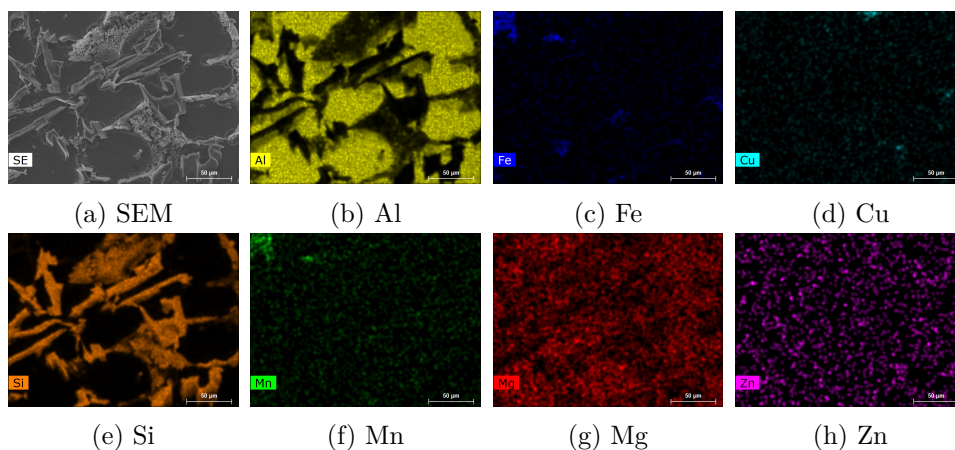
Figure 4.3: Paineil comparativo SEM-EDS em disposição compacta de 2x4.
