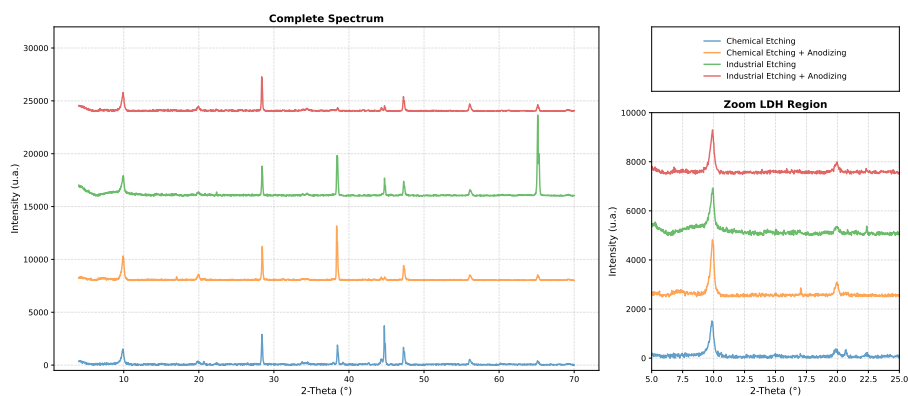
Figure 4.7: Padrões de difração de raios X (XRD) originais e com zoom na região intercalar dos LDHs após remoção da linha de base.
