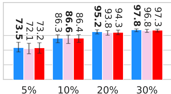
MLP
