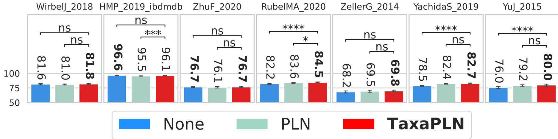
XGBoost AUPRC (%)
