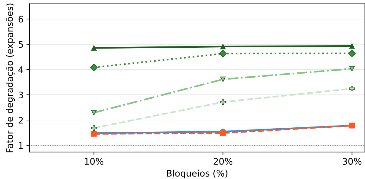
Fator de degradação de expansões por tipo de bloqueio
