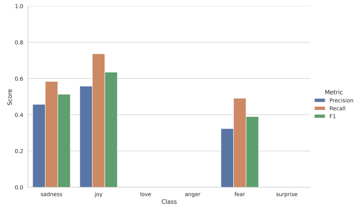
Figura 8: Rappresentazione grafica delle metriche in configurazione One-Shot
