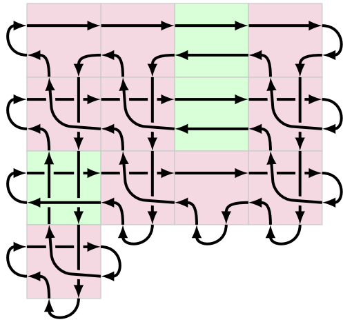
L''_{v,w}
