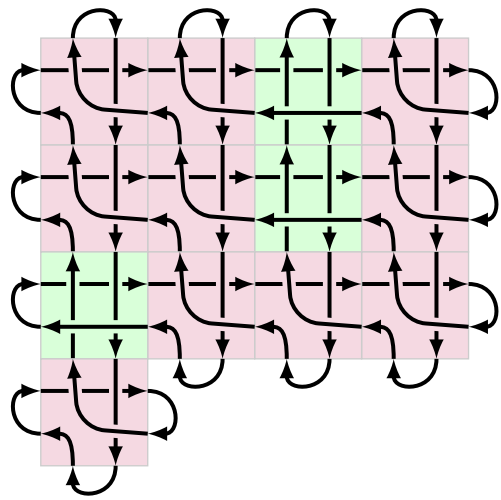
L'_{v,w}
