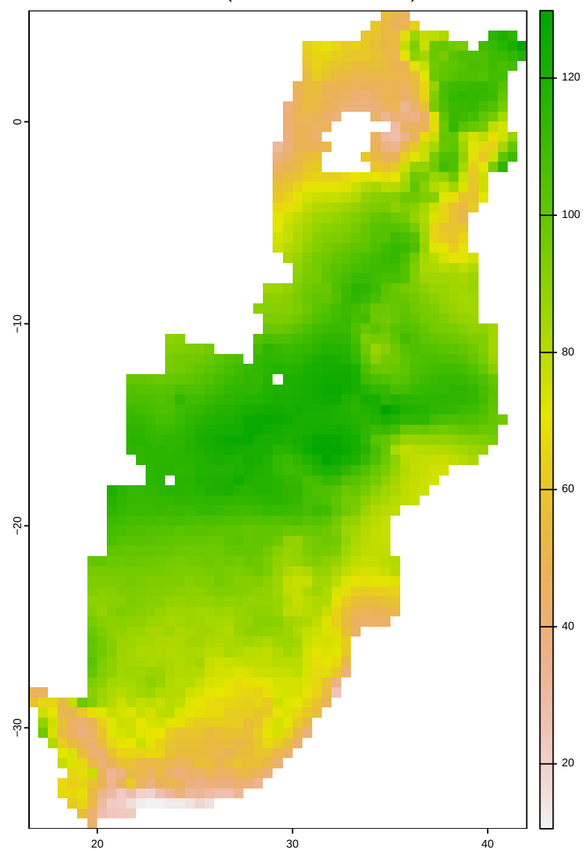
P of warmest qtr (mm qtr -1 )
