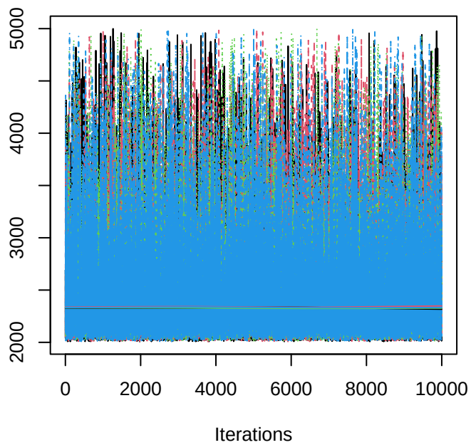
a[18]
