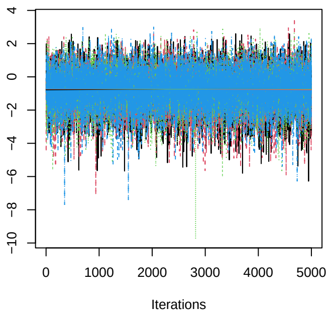
\nabla[18]
