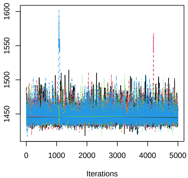
a[18]
