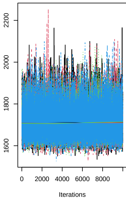
a[24]
