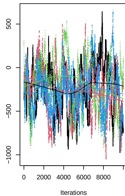
beta3
