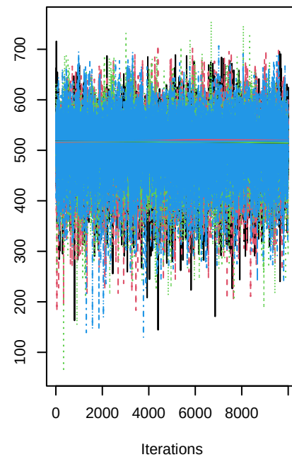
b[24]
