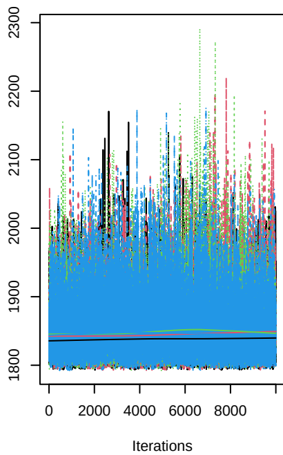
a[24]
