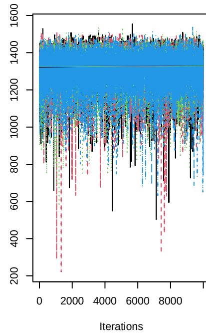
b[24]
