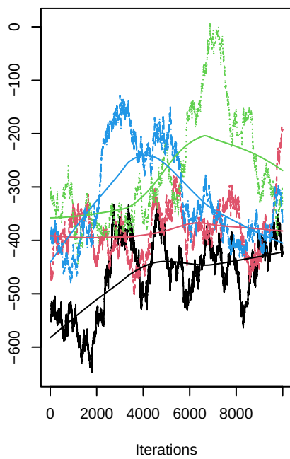
beta1
