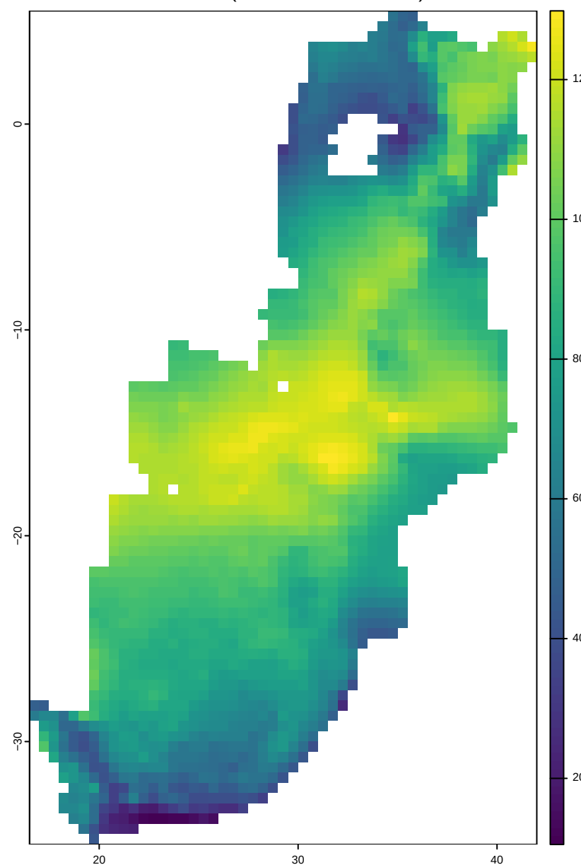
P of warmest qtr (mm qtr -1 )
