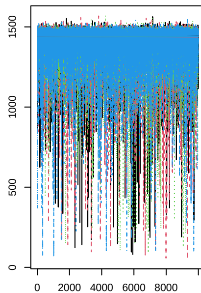
b[24]
