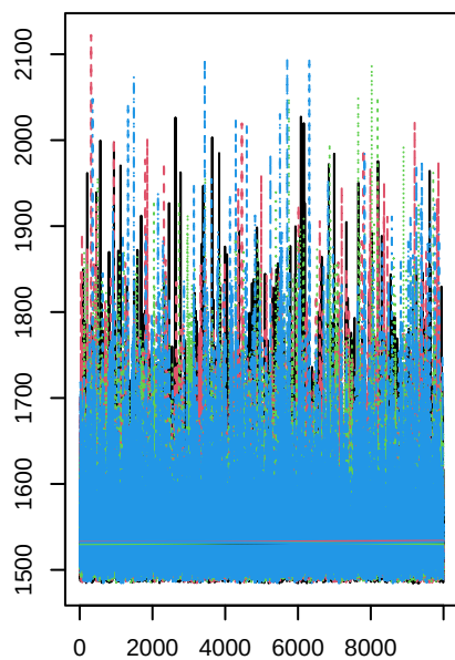
a[24]
