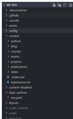
Рис. 1: Структура проекта персонального сайта
