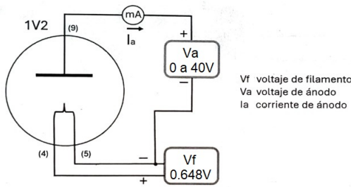
Figura 2. Diagrama del arreglo experimental
