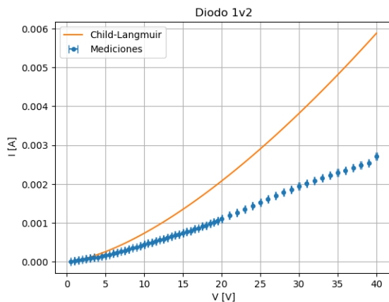
Figura 3. Datos obtenidos para los voltajes registrados. La línea continua representa el valor esperado a partir de la Ley de Child-Langmuir
