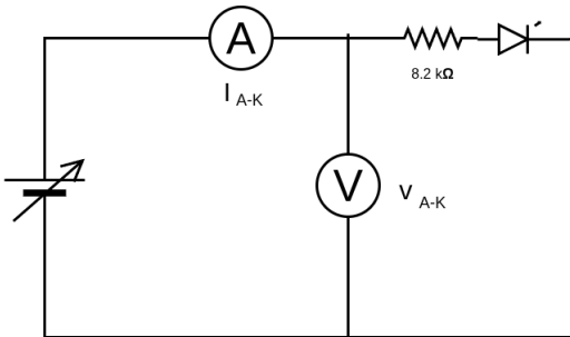
Figura 2. Circuito para medir la corriente y voltaje de un LED con una resistencia de 8,2\text{ k}\Omega conectados a una fuente variable.
