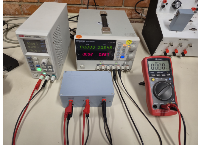
Figura 1. Arreglo experimental usando un diodo al vacío 1v2
