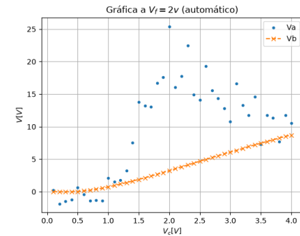
Figura 7. Gráfica del voltaje del ánodo y del voltaje de la rejilla-blindaje registradas por el software del laboratorio contra el voltaje del cátodo a un voltaje fuente de 2\text{ V} .
