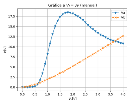
Figura 5. Gráfica del voltaje del ánodo y del voltaje de la rejilla-blindaje registradas por el multímetro contra el voltaje del cátodo a un voltaje fuente de 3\text{ V} .
