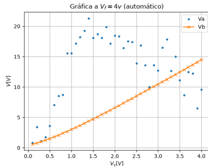
Figura 9. Gráfica del voltaje del ánodo y del voltaje de la rejilla-blindaje registradas por el software del laboratorio contra el voltaje del cátodo a un voltaje fuente de 4\text{ V} .
