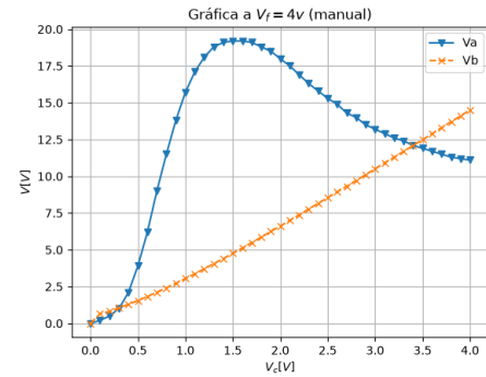
Figura 6. Gráfica del voltaje del ánodo y del voltaje de la rejilla-blindaje registradas por el multímetro contra el voltaje del cátodo a un voltaje fuente de 4\text{ V} .
