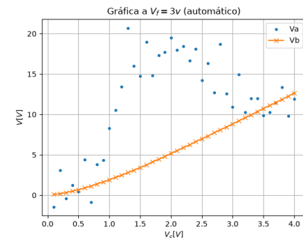
Figura 8. Gráfica del voltaje del ánodo y del voltaje de la rejilla-blindaje registradas por el software del laboratorio contra el voltaje del cátodo a un voltaje fuente de 3\text{ V} .
