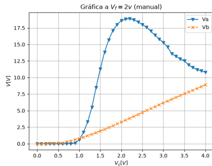
Figura 4. Gráfica del voltaje del ánodo y del voltaje de la rejilla-blindaje registradas por el multímetro contra el voltaje del cátodo a un voltaje fuente de 2\text{ V} .
