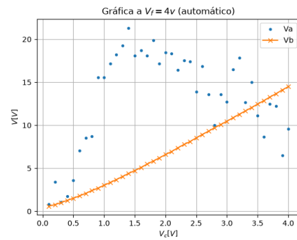
Figura 8. Gráfica del voltaje del ánodo y del voltaje de la rejilla-blindaje registradas por el software del laboratorio contra el voltaje del cátodo a un voltaje fuente de 4 V.
