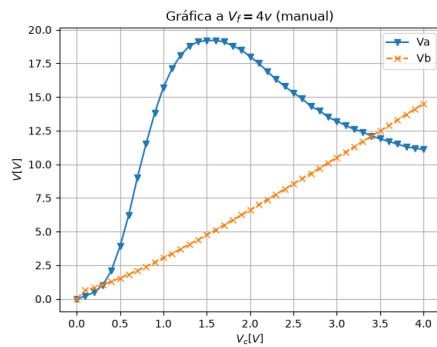
Figura 5. Gráfica del voltaje del ánodo y del voltaje de la rejilla-blindaje registradas por el multímetro contra el voltaje del cátodo a un voltaje fuente de 4 V.
