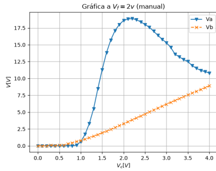
Figura 3. Gráfica del voltaje del ánodo y del voltaje de la rejilla-blindaje registradas por el multímetro contra el voltaje del cátodo a un voltaje fuente de 2 V.
