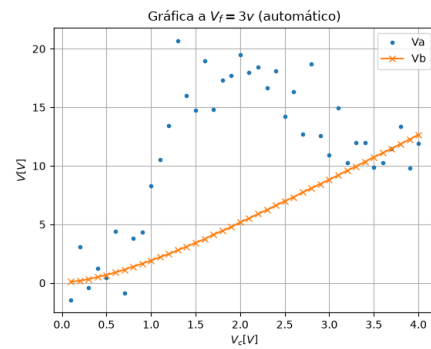
Figura 7. Gráfica del voltaje del ánodo y del voltaje de la rejilla-blindaje registradas por el software del laboratorio contra el voltaje del cátodo a un voltaje fuente de 3 V.
