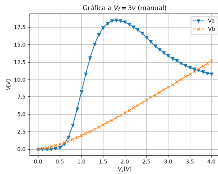
Figura 4. Gráfica del voltaje del ánodo y del voltaje de la rejilla-blindaje registradas por el multímetro contra el voltaje del cátodo a un voltaje fuente de 3 V.
