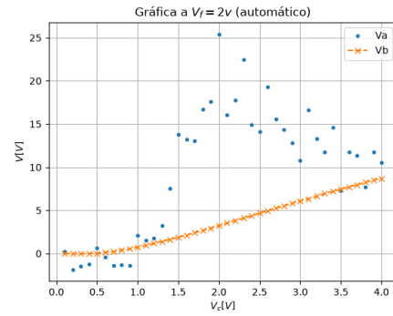
Figura 6. Gráfica del voltaje del ánodo y del voltaje de la rejilla-blindaje registradas por el software del laboratorio contra el voltaje del cátodo a un voltaje fuente de 2 V.
