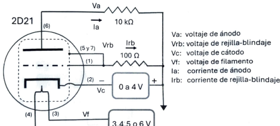
Figura 1. Diagrama de conexión interna del módulo con el bulbo 2D21.
