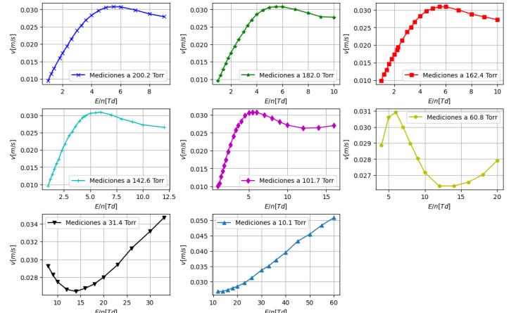
Figura 5. Gráficas de campo eléctrico reducido contra velocidad de deriva a diferentes presiones
