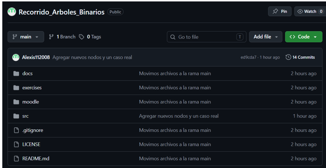
Ilustración 1. Repositorio Recorrido_Arboles_Binarios
