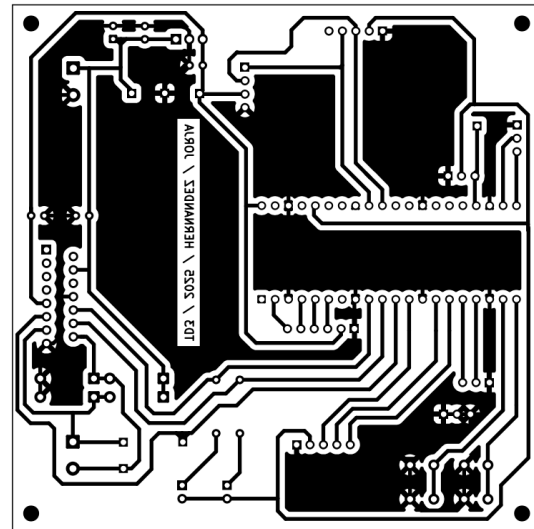
Fig. 9 Vista de las pistas del PCB
