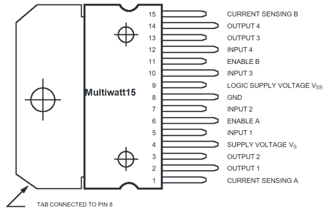
Fig. 3 Pinout L298N
