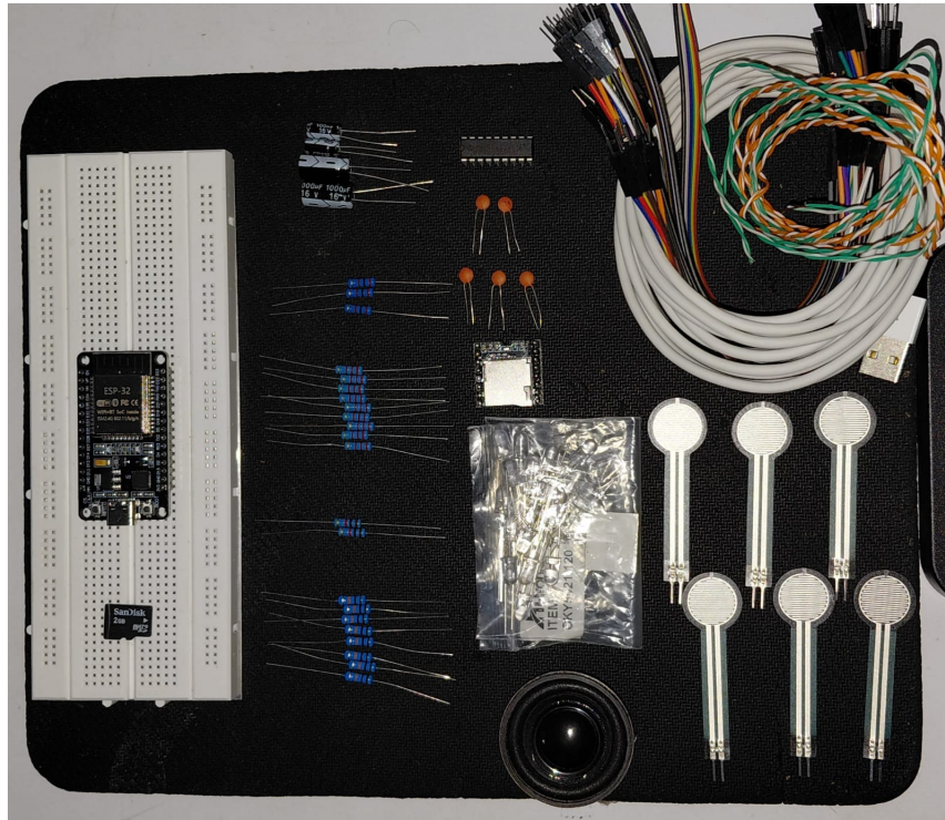
Figura 1: Inventario de componentes del prototipo: placa de prototipado con el módulo ESP32, arreglo de conmutación, módulo de audio con tarjeta microSD, parlante, condensadores, resistencias, diodos emisores de luz, cableado y los seis sensores de presión resistivos (abajo a la derecha).
