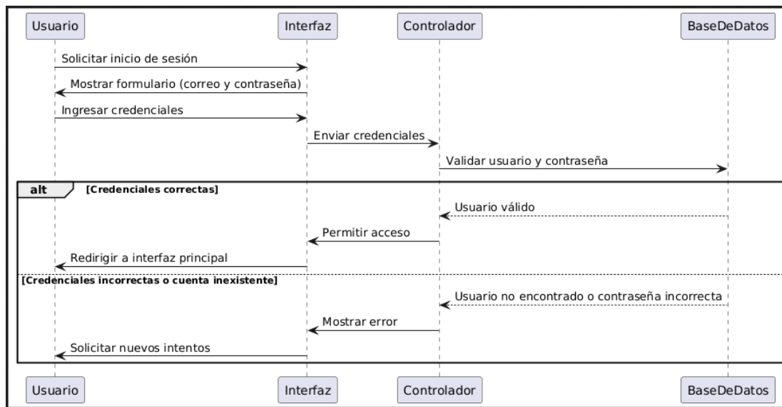
Figura 22: Diagrama de secuencia iniciar sesión
