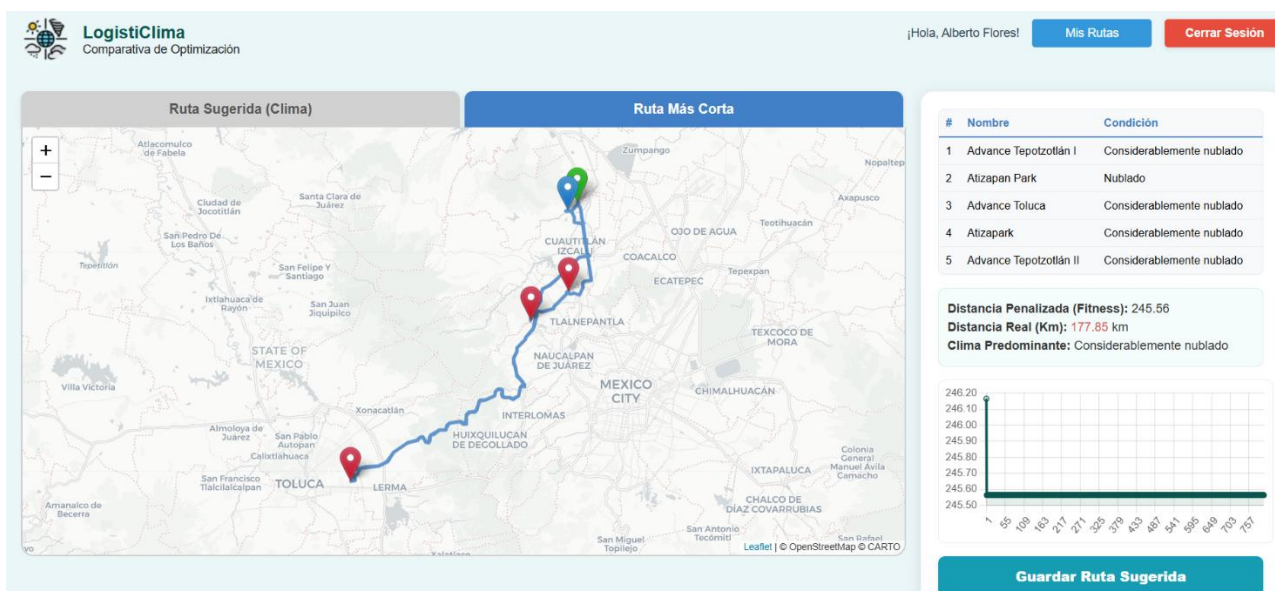
Figura 72: Vista del mapa con el trazado de la ruta sin penalizar
