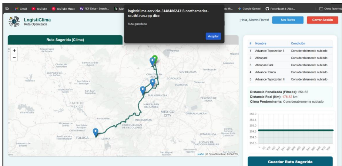
Figura 91: Guardar la ruta después de generar el resultado
