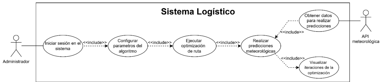
Figura 11: Diagrama de casos de uso para Administrador
