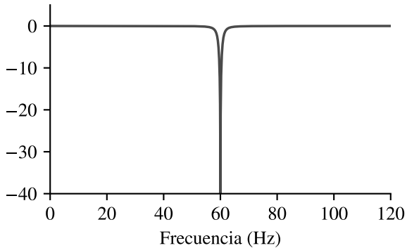
(b) Filtro notch en 60 Hz ( Q = 30 )
