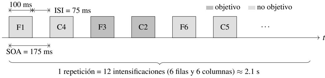
Figura 2.8: Parámetros de estimulación del P300 Speller con los valores de la base de datos II de la competencia BCI III (F = fila, C = columna). Elaboración propia con base en [14].
