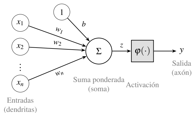
Figura 2.14: Modelo de la neurona artificial y su analogía con la neurona biológica. Elaboración propia con base en [47].
