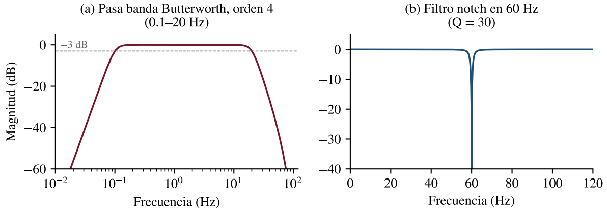
Figura 2.10: Respuesta en magnitud de (a) un filtro pasa banda Butterworth de cuarto orden entre 0.1 y 20 Hz y (b) un filtro notch en 60 Hz, para f_s = 240 Hz. Elaboración propia.
