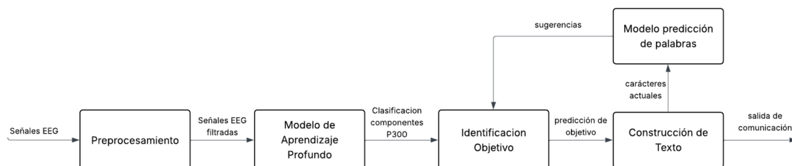
Figura 3.1: Arquitectura del sistema. Elaboración propia.
