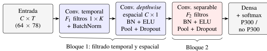
Figura 2.16: Arquitectura general de EEGNet. Elaboración propia con base en [49].
