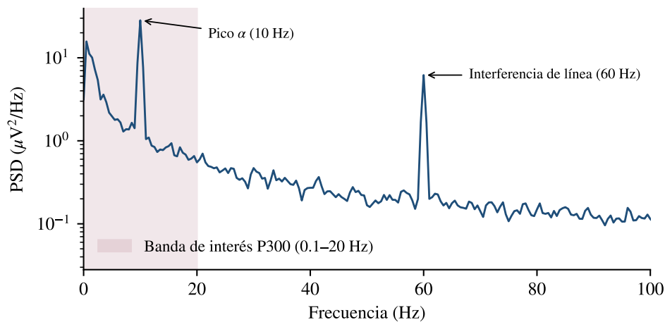
Figura 2.9: Densidad espectral de potencia estimada con el método de Welch para una señal de EEG sintética. Elaboración propia.
