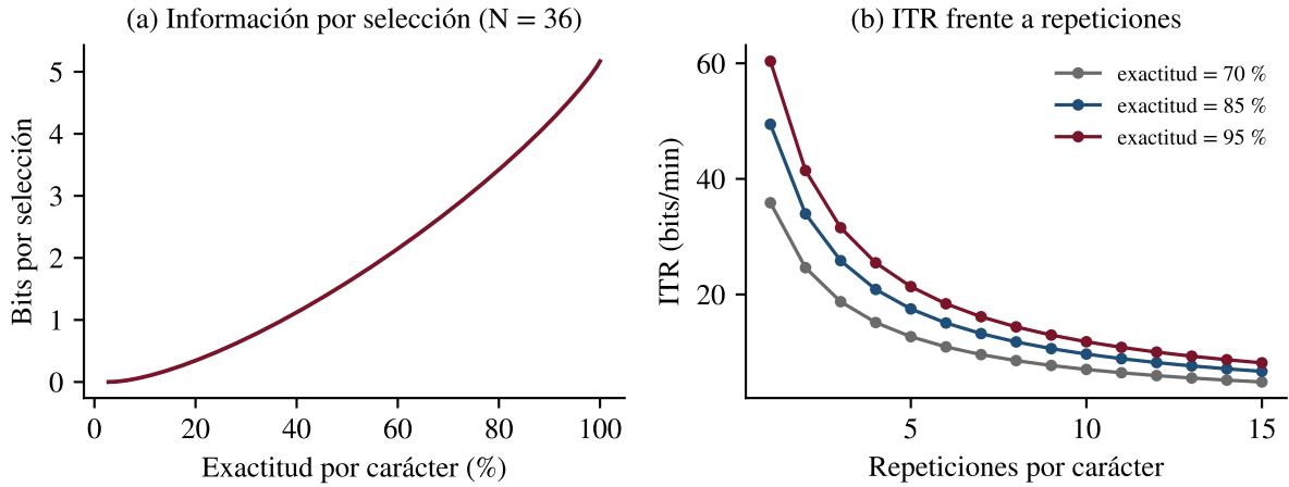
Figura 2.19: (a) Bits por selección en función de la exactitud para N = 36 según la Ecuación (2.10). (b) ITR teórica en función del número de repeticiones para tres niveles de exactitud, considerando 175 ms por intensificación y 2.5 s entre caracteres. Elaboración propia.
