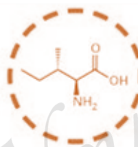
Isoleucina
