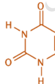
Uracilo
