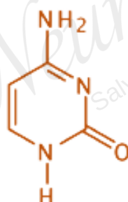
Citosina
