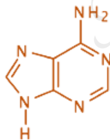
Adenina
