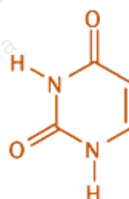
Uracilo
