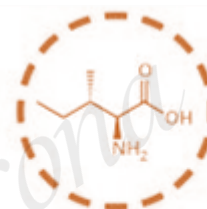
Isoleucina
