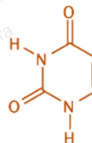
Uracilo
