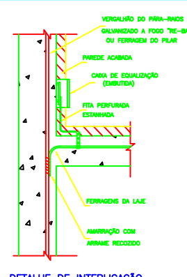
DETALHE DE INTERLIGAÇÃO DA CAIXA DE IGUALIZAÇÃO
