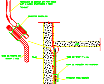
DETALHE DE AMARRAÇÃO DO VERGALHO DE DESCIDA COM O VERGALHO HORIZONTAL
