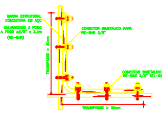
DETALHE DE AMARRAÇÃO DO VERGALHO DE DESCIDA COM O VERGALHO HORIZONTAL
