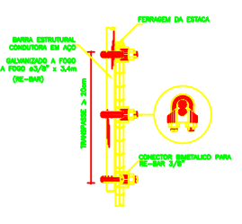
DETALHE DE ENLACE DO VERGALHO DE DESCIDA
