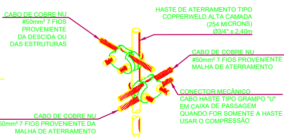
DETALHE DE ENLACE DO VERGALHO DE DESCIDA
