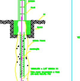
DETALHE DE ENLACE DO VERGALHO DE DESCIDA
