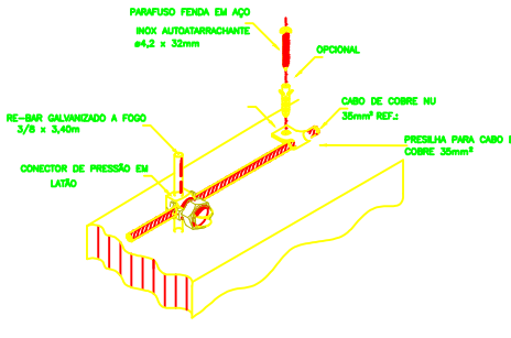
DETALHE DE FIXAÇÃO DO CABO DE COBRE E RE-BAR NA PLATIBANDA
