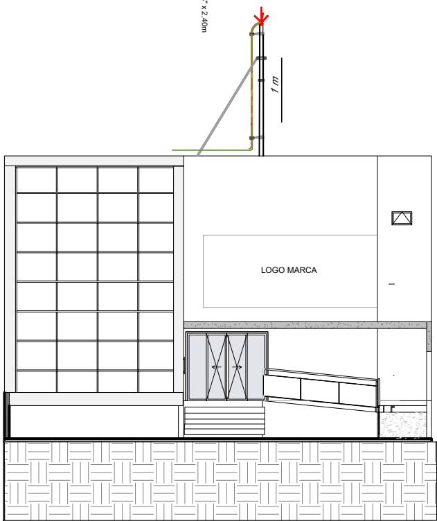
VISTA FACHADA PARA RAIOS
