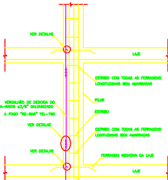
PE DIRETO GENÉRIO E AMARRAÇÕES
