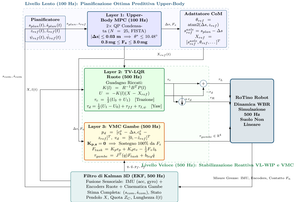
Figura 2: Schema a blocchi dell'architettura gerarchica disaccoppiata MPC + TV-LQR + VMC (rotino_mpc) con disaccoppiamento multi-frequenza 100 Hz / 500 Hz, ottimizzatore QP FISTA, controllo LQR con tabella di Riccati CARE e Filtro di Kalman 3D.
