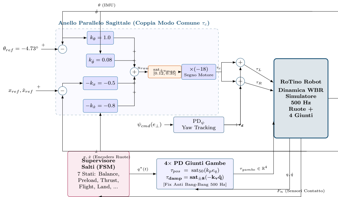
Figura 1: Schema a blocchi dettagliato del controllore PID ( rotino_pid ) con 4 anelli sagittali paralleli, anello di imbardata, supervisore dei salti FSM e PD di giunto anti-bang-bang.
