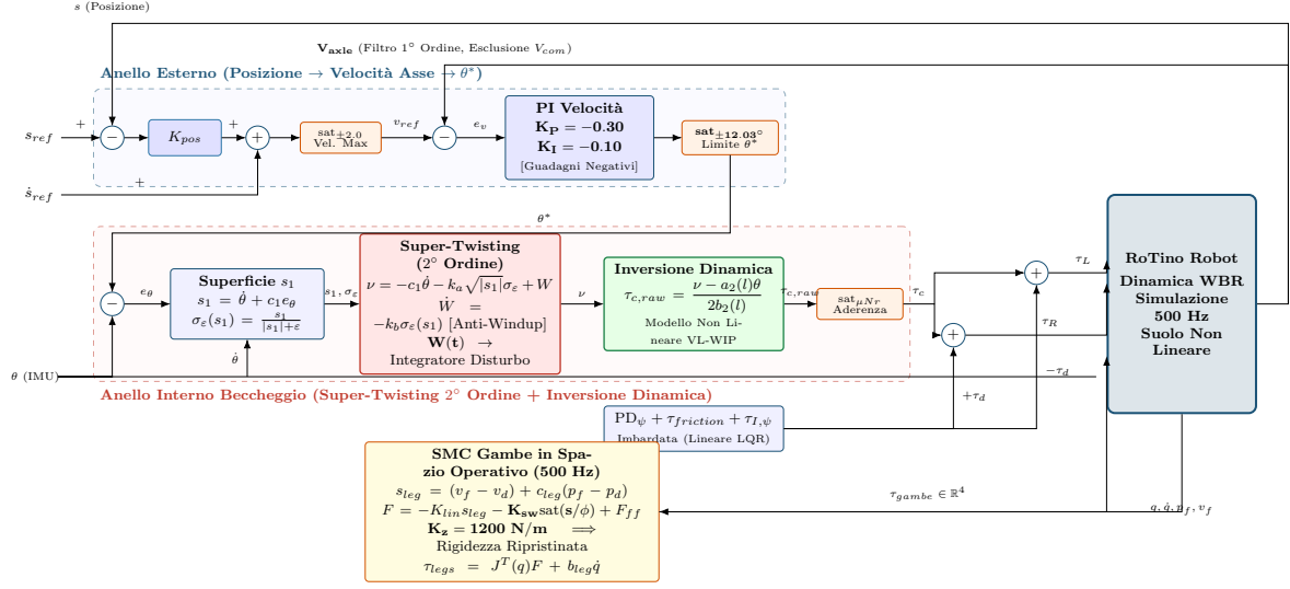
Figura 3: Schema a blocchi dell'architettura di controllo in cascata Sliding Mode ( rotino.smc ) con regolazione di velocità ad asse isolato, anello di beccheggio Super-Twisting del 2° ordine, inversione dinamica VL-WIP e SMC nello spazio operativo delle gambe.
