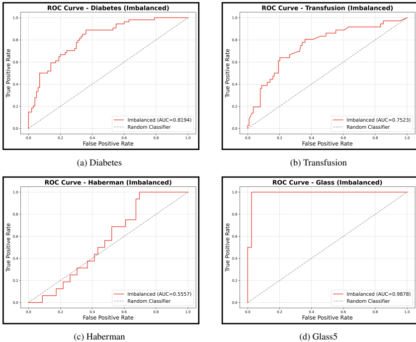
Gambar 4.2 Kurva ROC Baseline pada Data Tidak Seimbang
