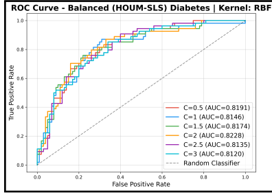
(b) Kernel RBF
