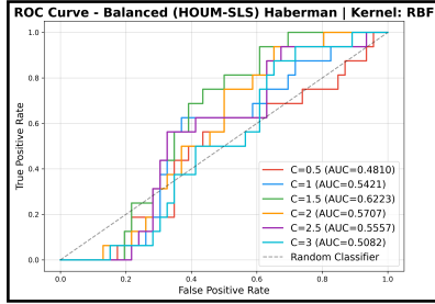
(b) Kernel RBF
