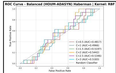
(b) Kernel RBF
