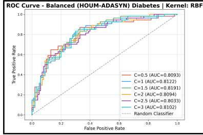
(b) Kernel RBF
