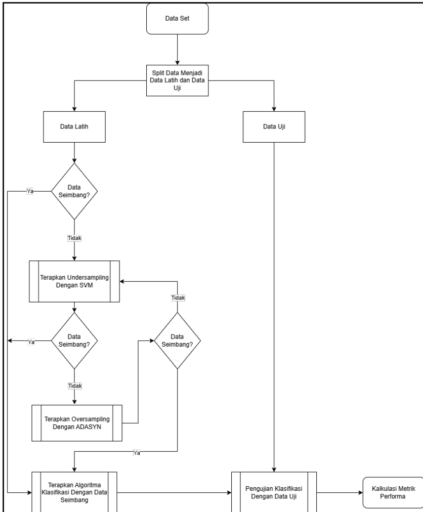
Gambar 2.4 Alur Kerja Metode HOUM
