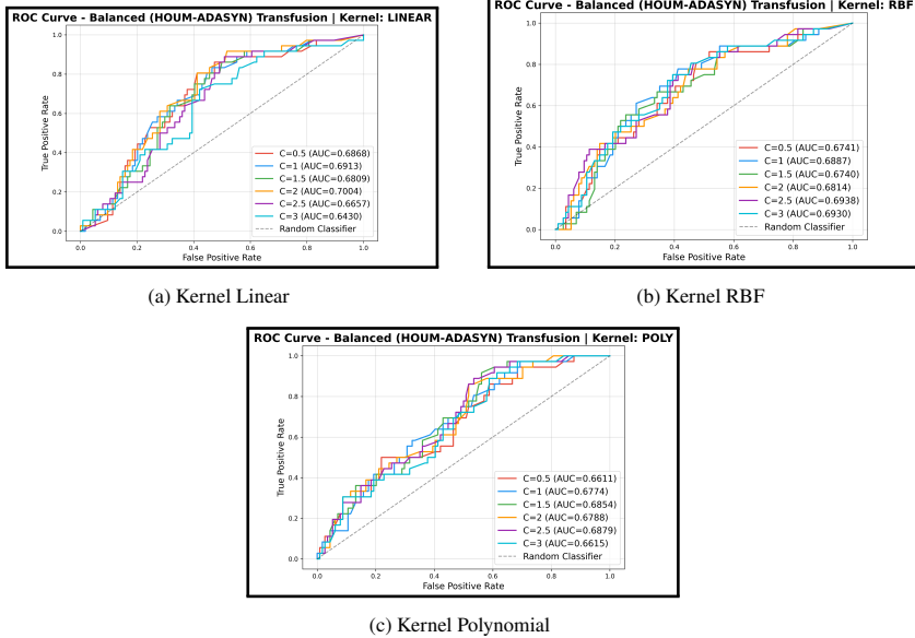
Gambar 4.9 Kurva ROC HOUM-ADASYN pada Dataset Transfusion
