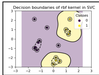
(b) Kernel RBF
