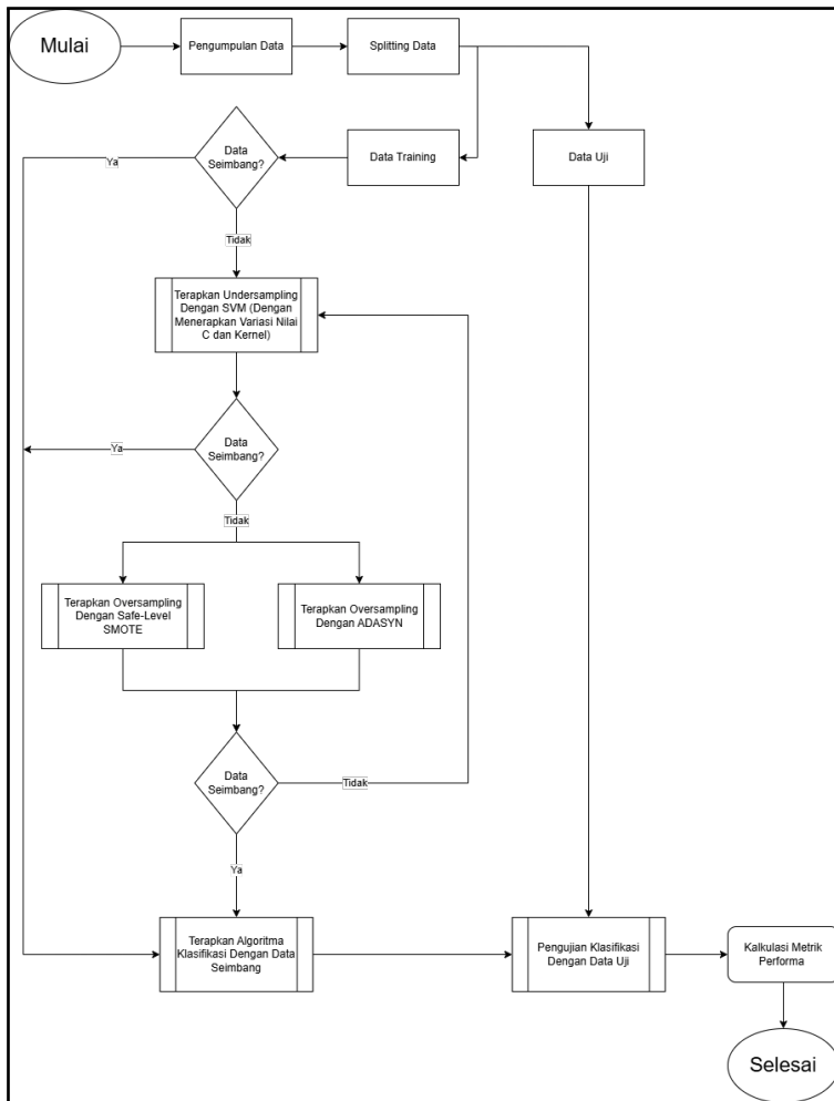
Gambar 3.2 Alur Implementasi Metode HOU
