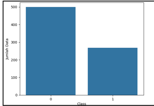
Gambar 2.1 Ilustrasi Distribusi Data Tidak Seimbang
