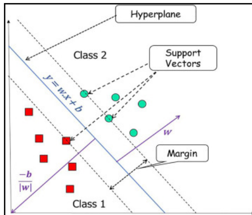
Gambar 2.5 Ilustrasi SVM
