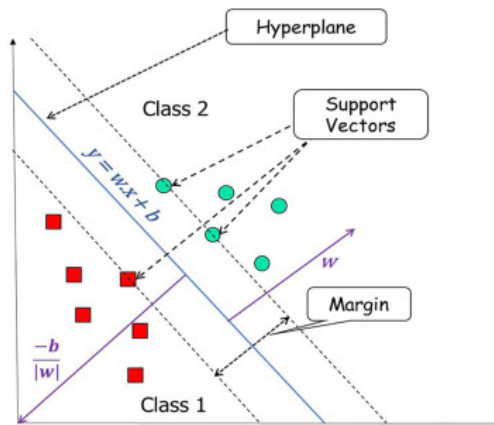
Gambar 2.5 Ilustrasi SVM
