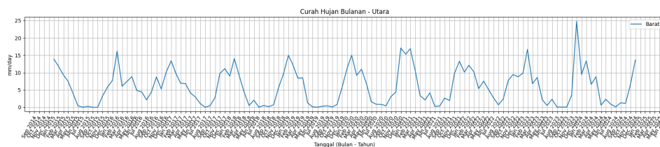
Gambar 4.5: Pola Curah Hujan Wilayah Utara
