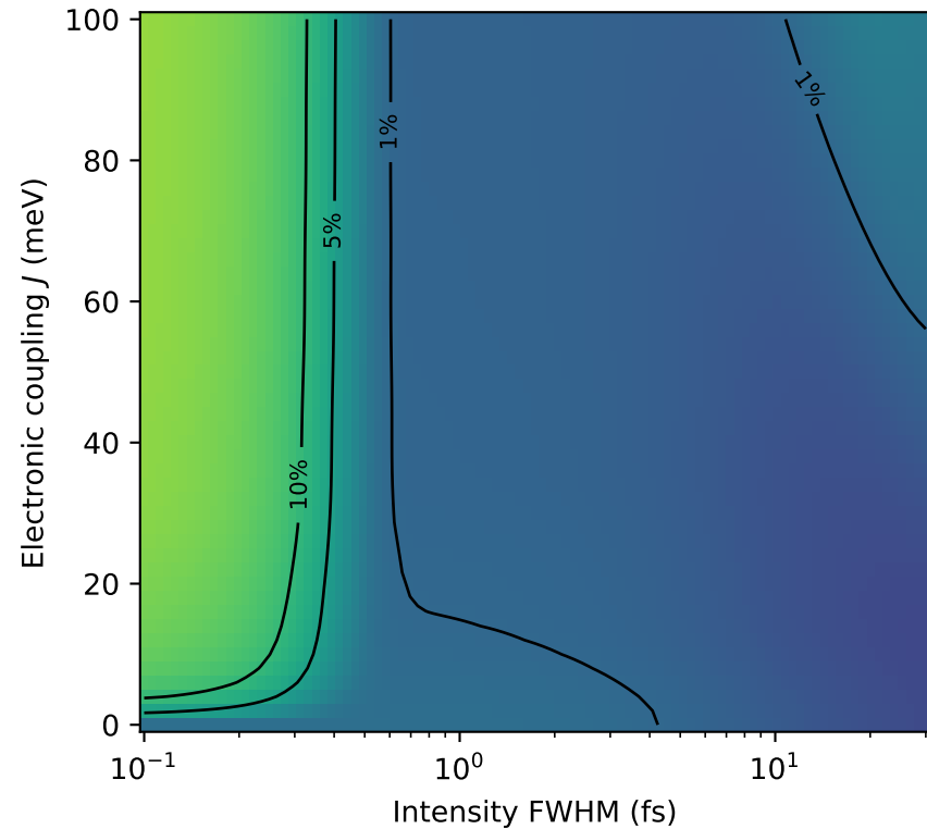
(a) RWA error: A - B
